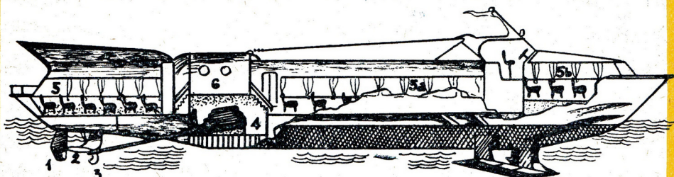
1. Руль. — 2. Заднее несущее крыло. — 3. Гребной винт. — 4. Двигатель — 5. а и б — Места для пассажиров. — 6. Передние несущие крылья. — 7. Кабина рулевого.
